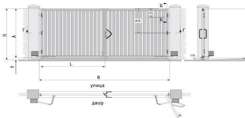
Внешний вид ограждающего устройства (габариты: 3890x1800мм)
